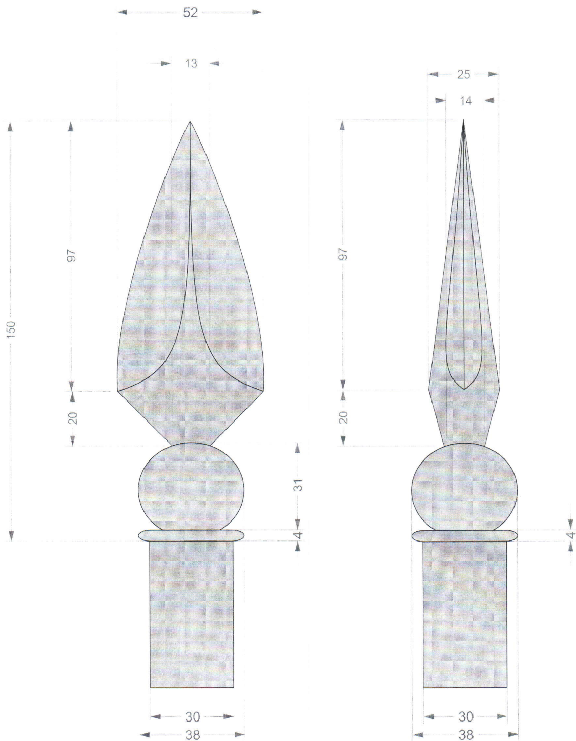
Слика 2. Изглед и димензије главе копља (у мм)
